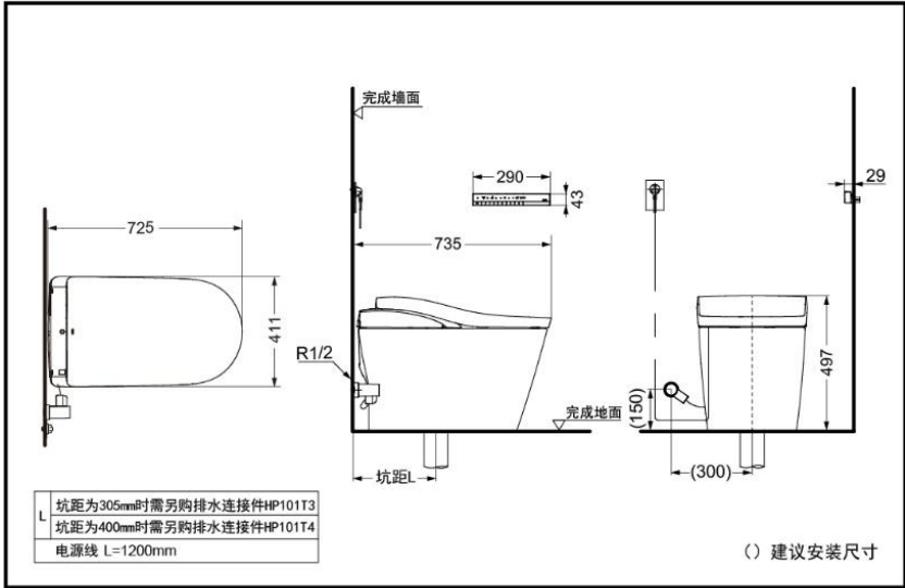
CES8G520GCN 诺锐斯特智能全自动一体型电子坐便器
