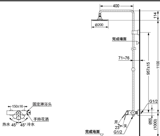
DM919CAR/DM919CA1 铜合金单柄双控淋浴柱
