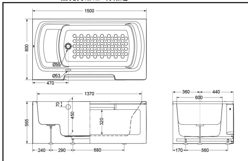
PAY1517LP 压克力浴缸 有裙边
