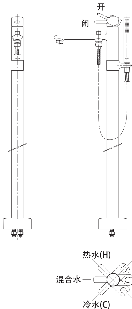
DM334CFN 铜合金立式单柄双控浴缸水嘴(可转换·带手持花洒)
