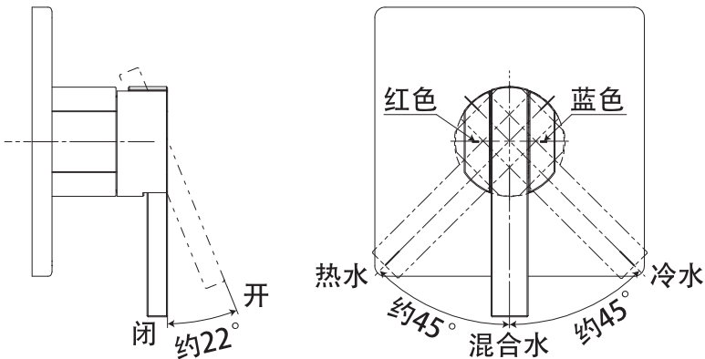
铜合金壁式单柄双控暗装水嘴面板（可转换）
