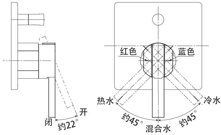
铜合金壁式单柄双控暗装水嘴面板（可转换）
