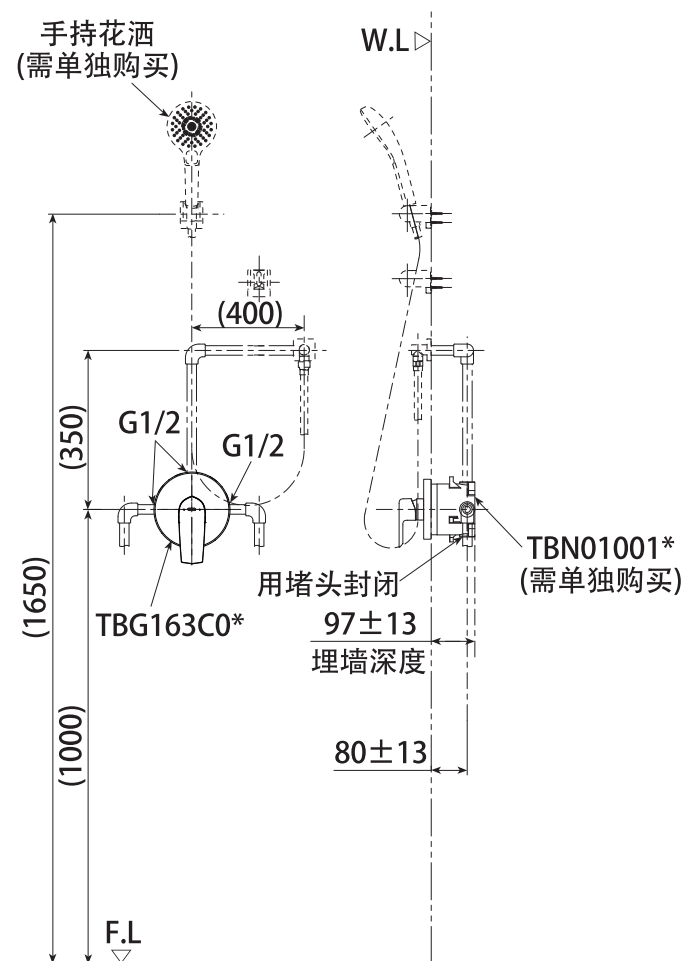
TBG163C0*铜合金壁式单柄双控暗装水嘴面板 与「TOTO」的其他产品配合示意图
