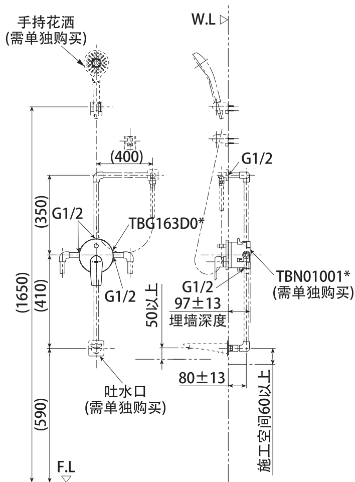
TBG163D0*铜合金壁式单柄双控暗装水嘴面板(可转换)与「TOTO」的其他产品配合示意图
