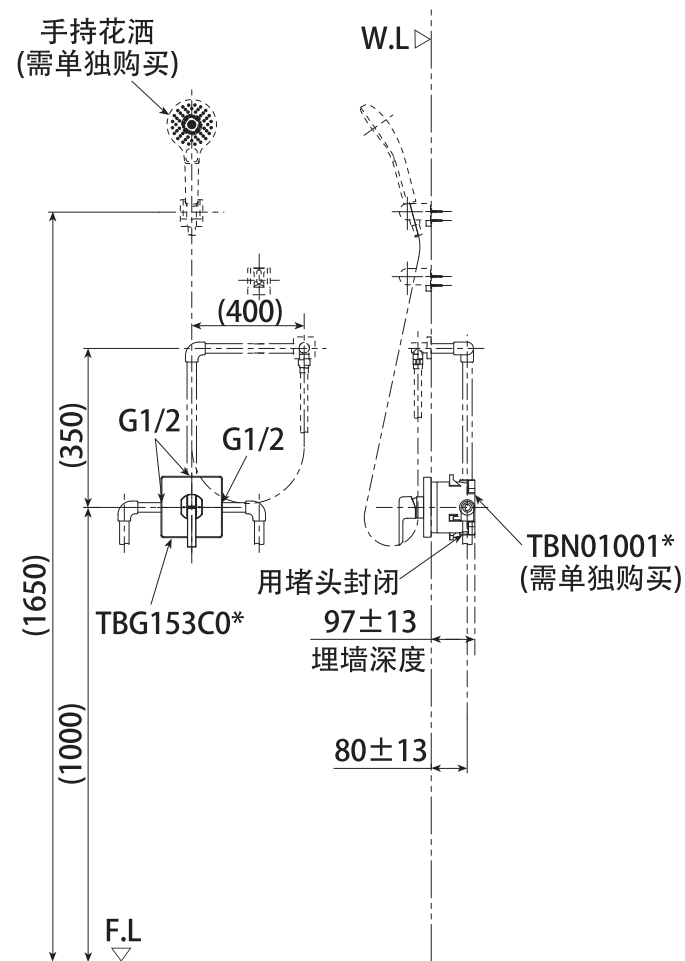
TBG153C0*铜合金壁式单柄双控暗装水嘴面板与「TOTO」的其他产品配合示意图
