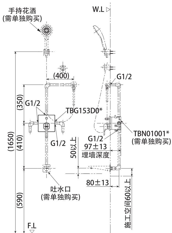
TBG153D0*铜合金壁式单柄双控暗装水嘴面板 (可转换) 与「TOTO」的其他产品配合示意图
