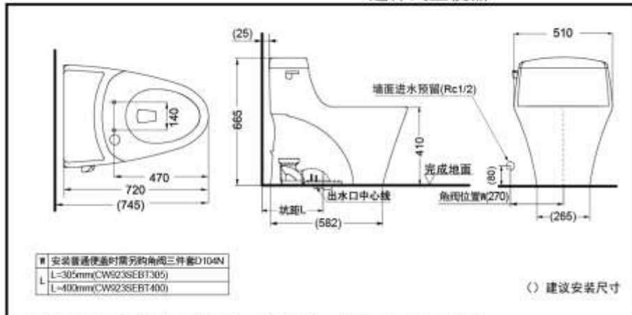
CW923SEBT305/CW923SEBT400 连体式坐便器
