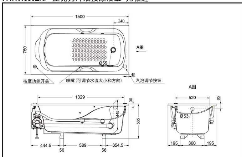
PAYK1550ZRHP PAYK1550ZRP 压克力冲浪按摩浴缸 无裙边
