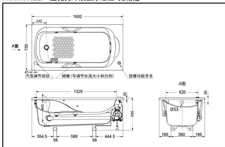
PAYK1550ZLHP PAYK1550ZLP 压克力冲浪按摩浴缸 无裙边
