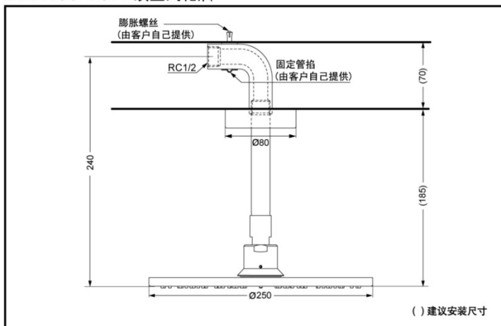
DBX133-1CA 顶置式花洒
