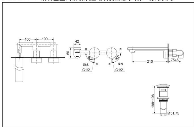
DLB203-1 铜合金壁式双柄双控暗装洗面器水嘴(CI现代系列)
