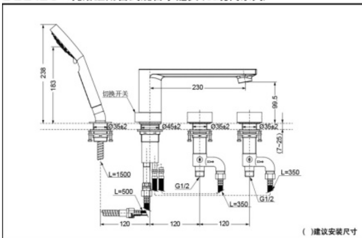
DB242C 4孔浴缸用台式混合水龙头 (CI现代系列)
