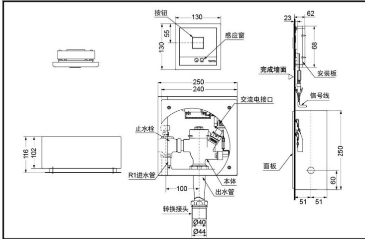
DCE602UE 感应式坐便器用自动冲洗阀(交流电型)
