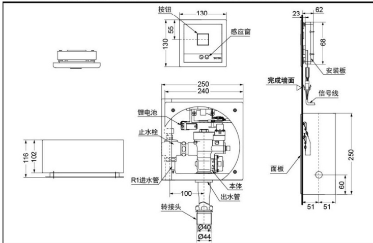
DCE602UH 感应式坐便器用自动冲洗阀(水力发电)
