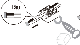
Power terminal block 电源端子台 電源端子台
