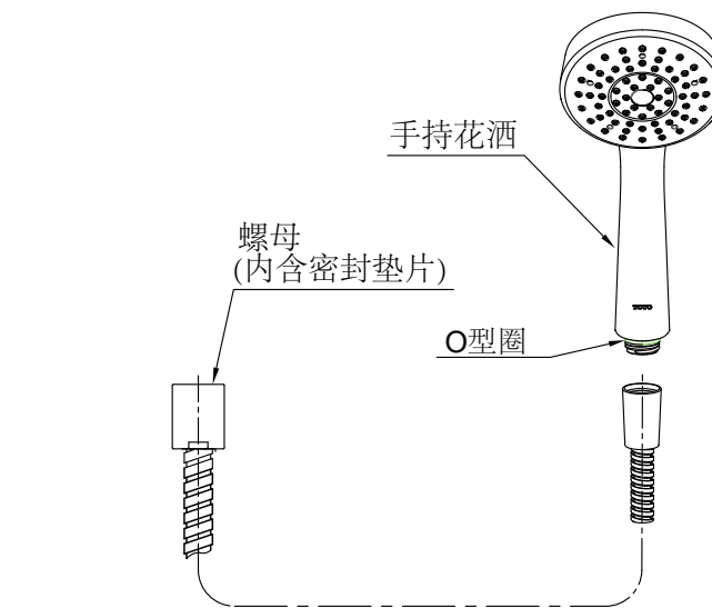
图2: 淋浴软管的安装
