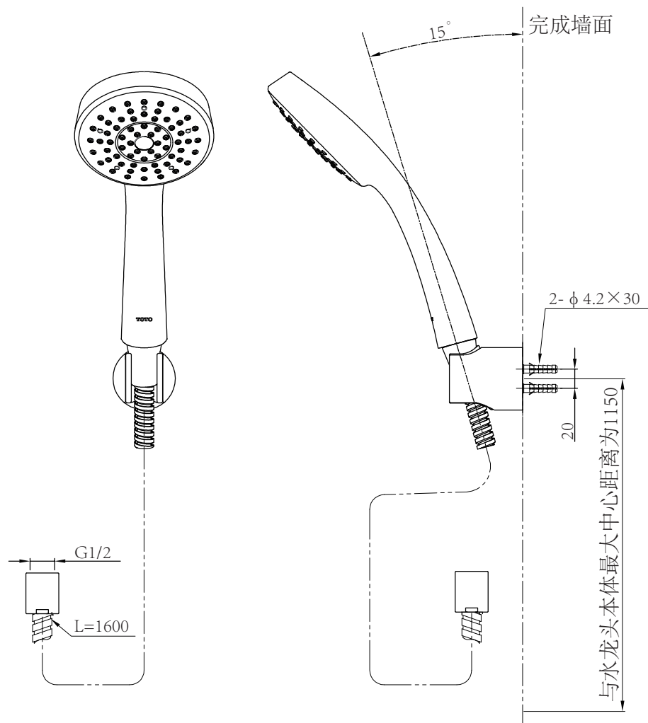
TBW01017*系列 单功能手持花洒 (浴室淋浴用)
