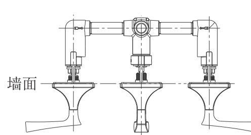
DB246AS手柄示意图
