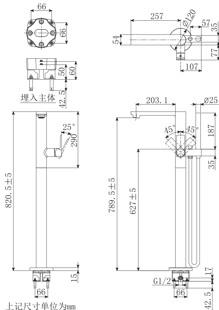
DM359CF 铜合金立式单柄双控浴缸水嘴(可转换·带手持花洒)
