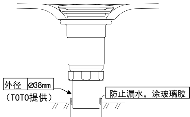
安装示意图
