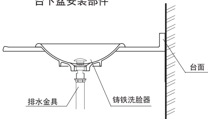
台上盆安装部件
