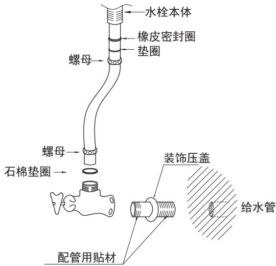
进水件安装详图
