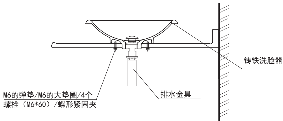
桌上盆安装部件
