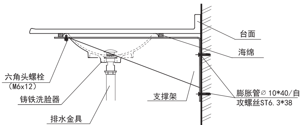
台下盆安装部件
