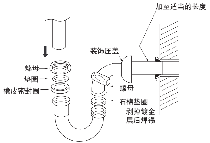
排水件安装详图
