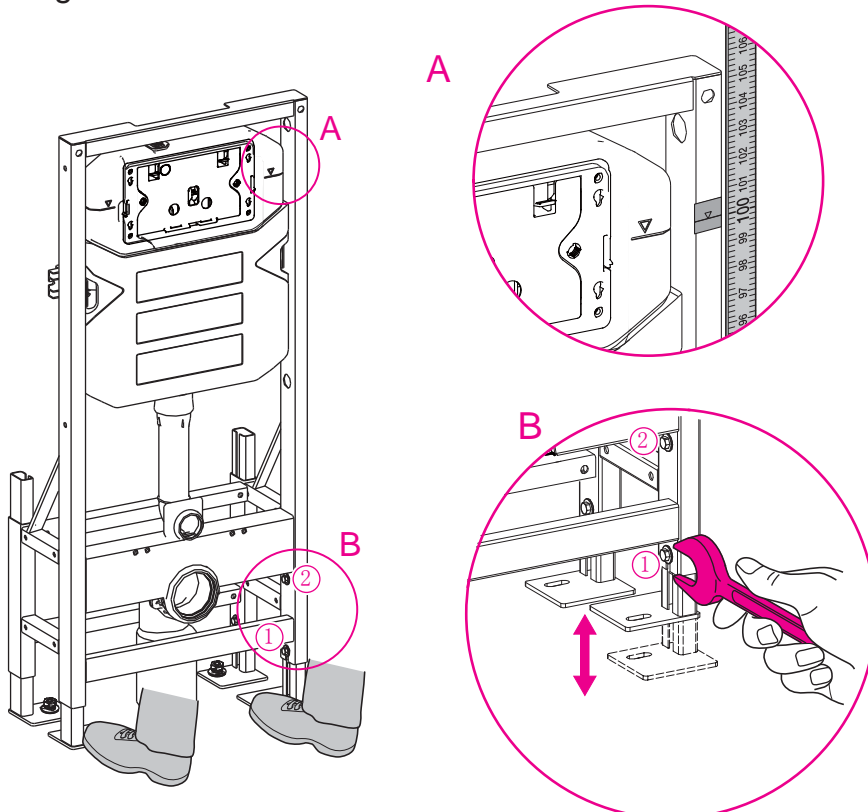
地面固定架。
