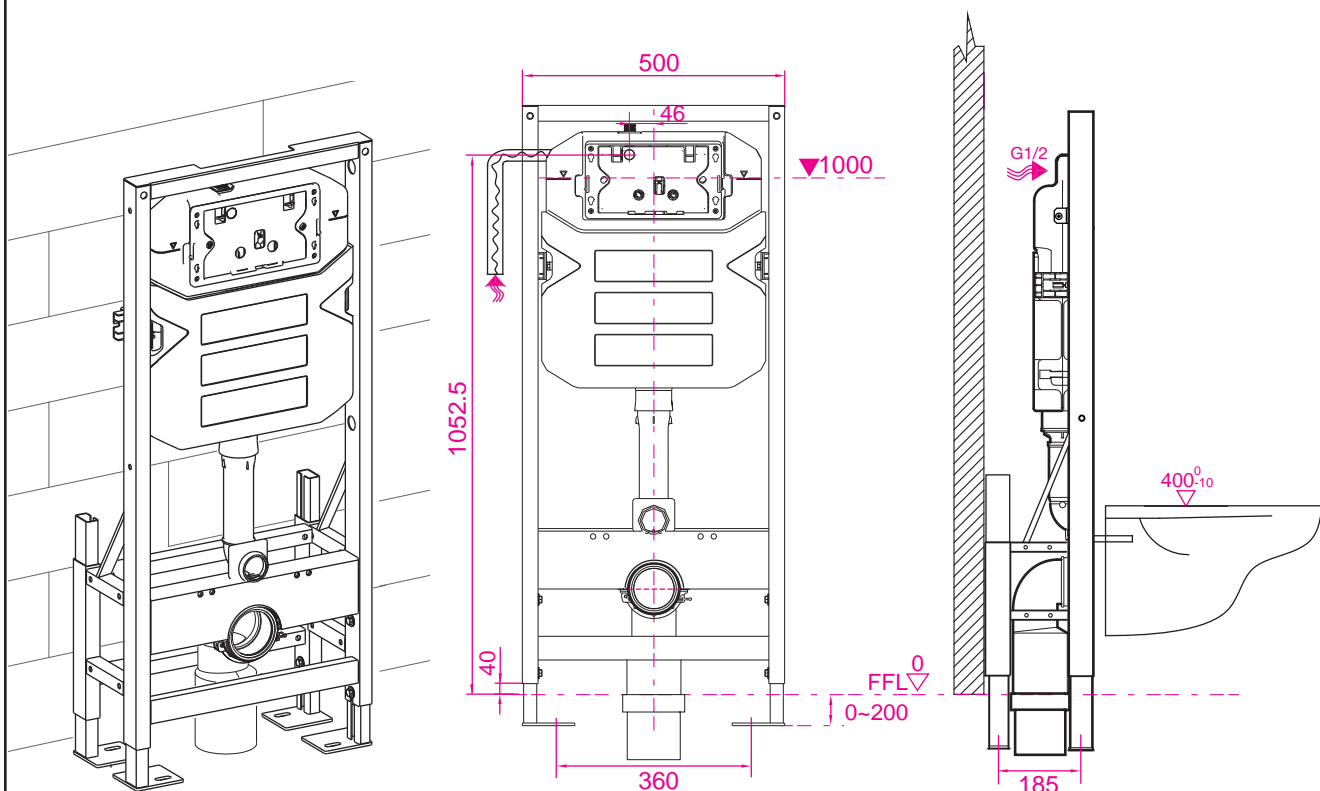
水箱后孔进水 Back inlet
