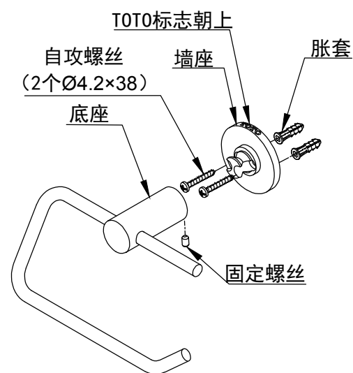
不带固定块 (DS727、DS727-1示例)
