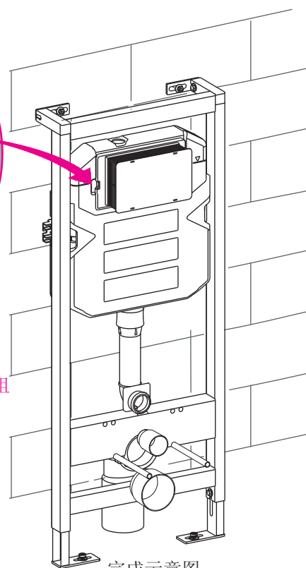
完成示意图 Sketch of installed frame
